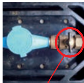
メーターボックス内止水栓 右に回すと水が止まります。
