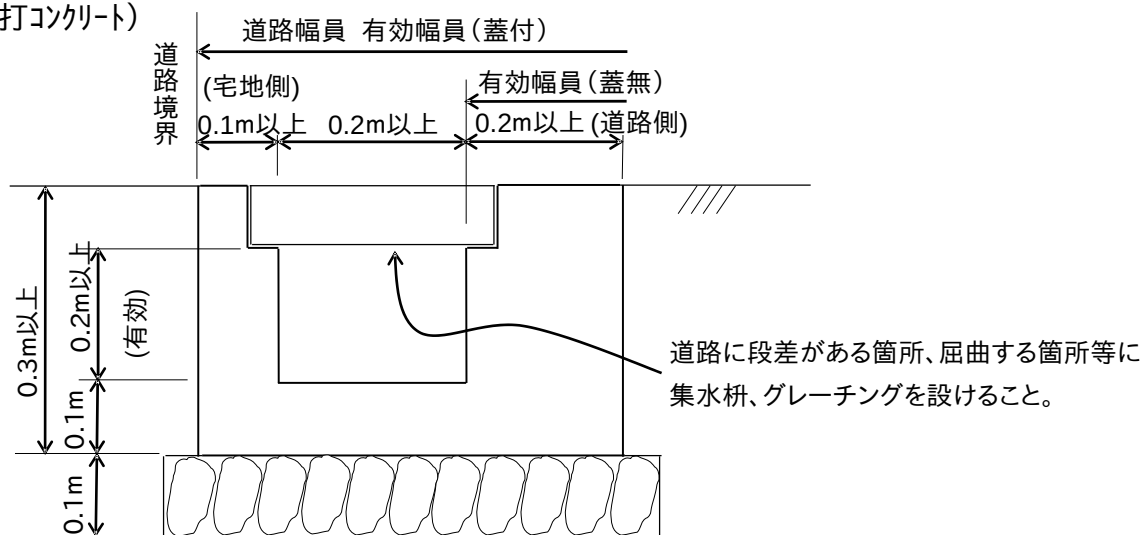
図11. 排水施設(標準図)
