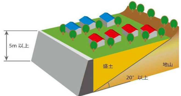
腹付け型大規模盛土造成地のイメージ
