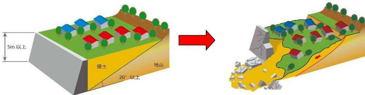
腹付け型大規模盛土造成地で発生する滑動崩落のイメージ
