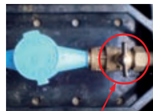
メーターボックス内止水栓 右に回すと水が止まります。
