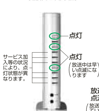
② ルーター (通信伝送中継装置)
